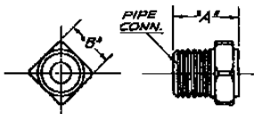
8400--PIPE PLUG
