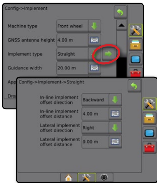
图 6-5: 偏移方向和距离
