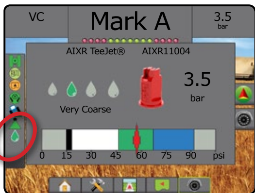
图 6-34: 液滴/压力状态
