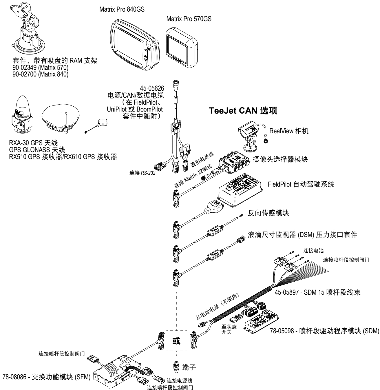
图 A-1: Matrix Pro GS
