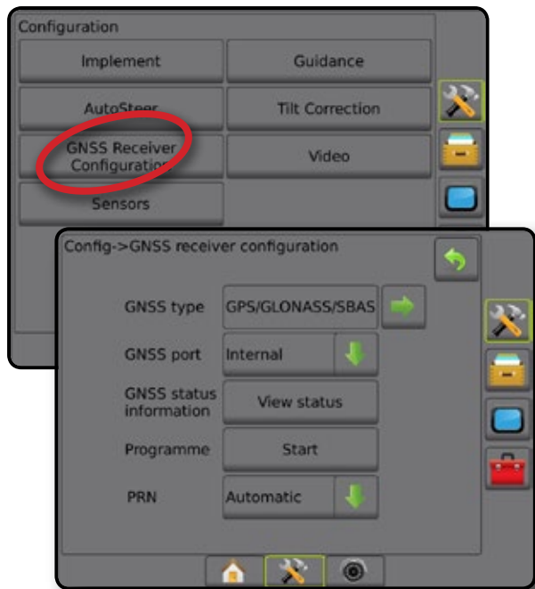
图 4-16: GNSS 接收器配置选项
