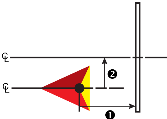
图 6-5: 偏移方向和距离
