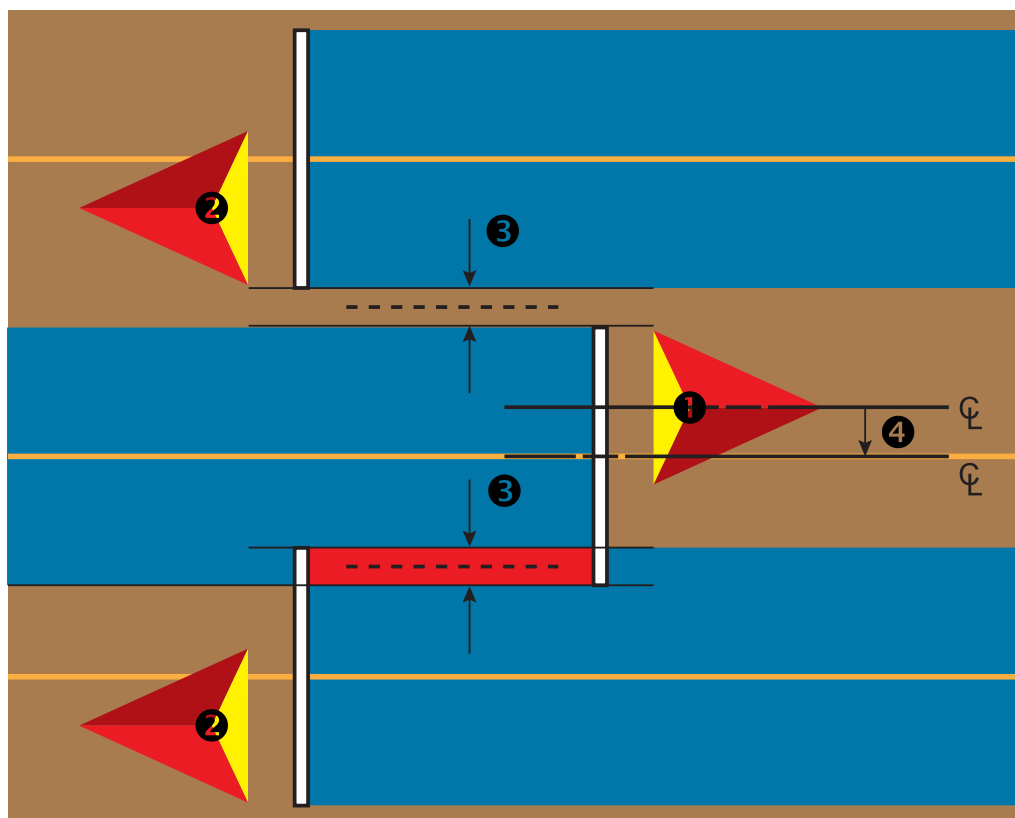
图 6-26: 横向执行区偏移距离和方向
