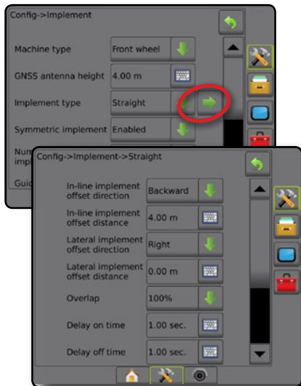
图 6-6: 多喷杆段
