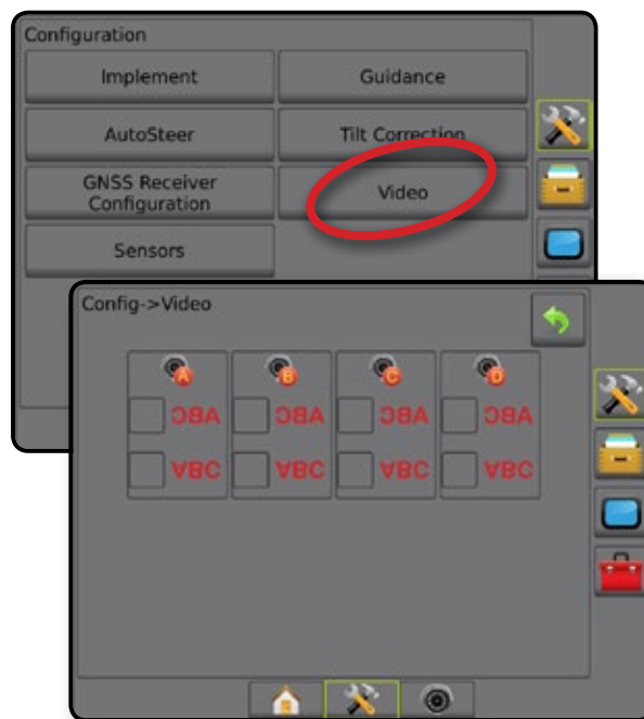
Bild 4-17: Video mit 4-Kanal-VSM-Optionen
