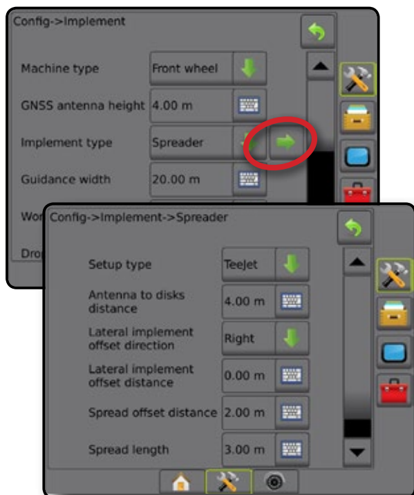
Bild 6-10: Abstände und Längen
