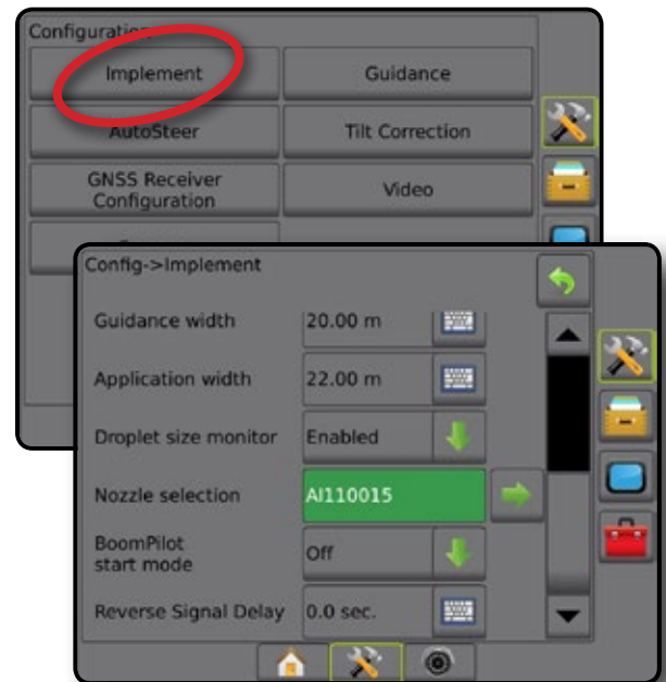
Bild 4-8: Tröpfchengrößenmonitor
