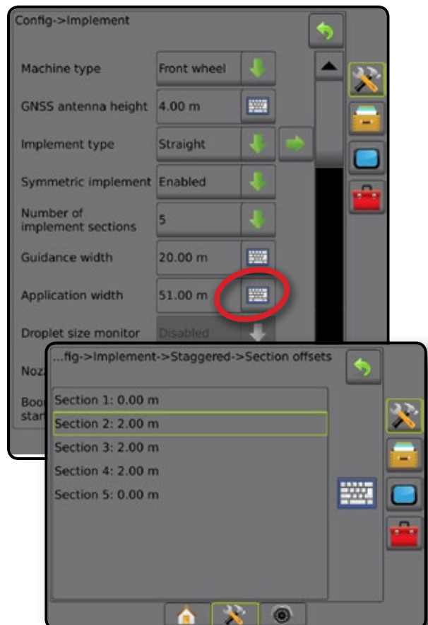
Bild 6-23: Mehrere Teilbreiten – Applikations- oder Behandlungsbreite
