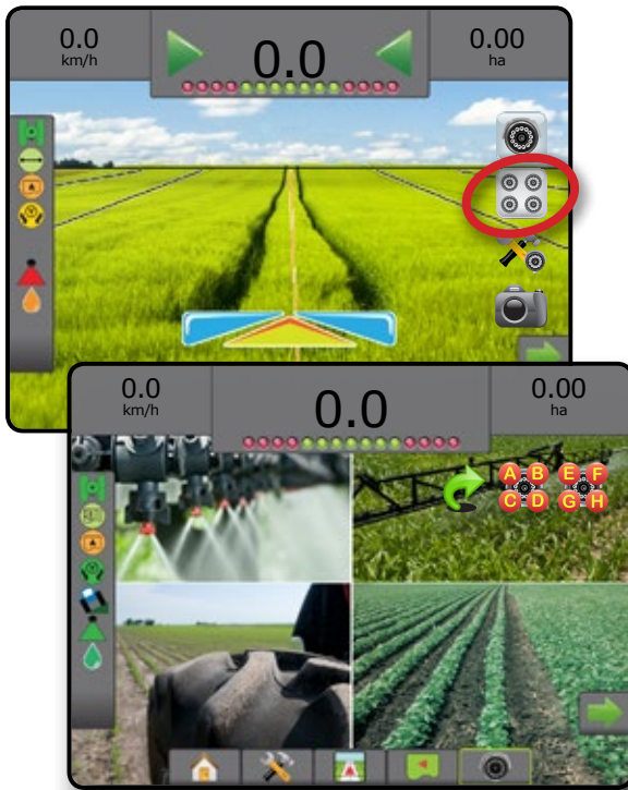
Bild 7-42: Auswahl der geteilten Bildschirmansicht über VSM
