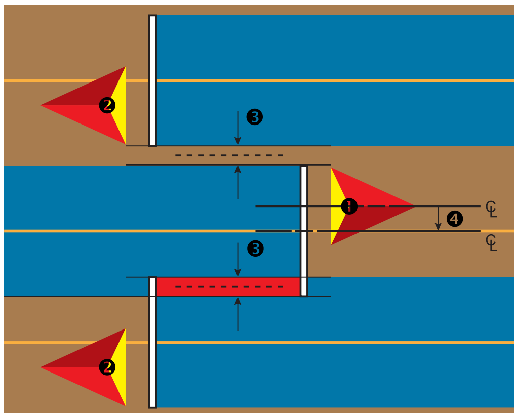
Figur 6-26: Sideværts redskab offset-distance og -retning
