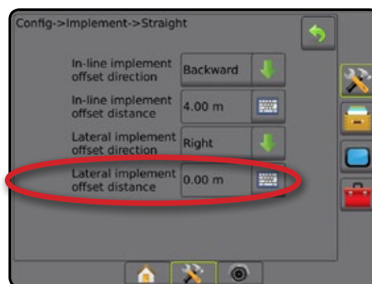
Figur 6-24: Sideværts redskab offset-distance
