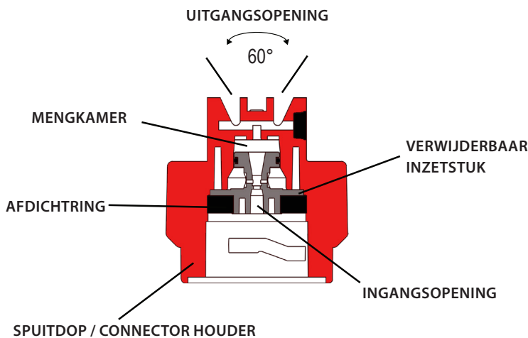
TTI60 DWARS AANZICHT
