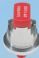
ДВУХФАКЕЛЬНЫЙ С ОГРАНИЧЕНИЕМ СНОСА (DGTJ60)
