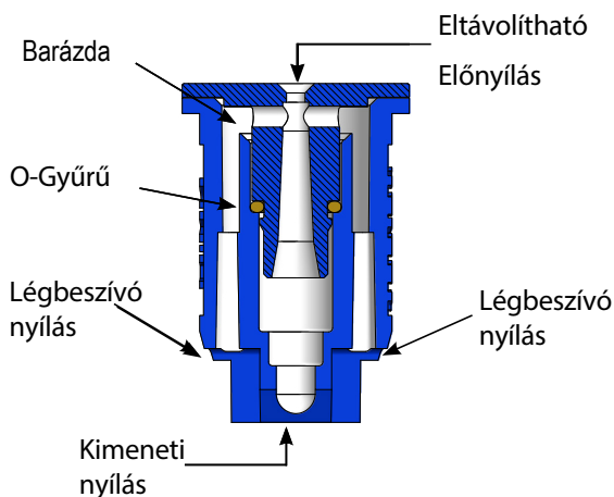
Szórófej AIXR110__VP (Keresztmetszeti nézet)
