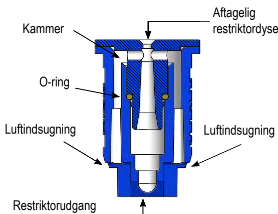
AIXR110 __ VP Dyse (Tværsnit)
