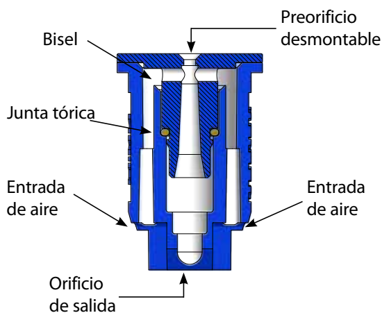
AIXR110__VP Boquilla (vista en corte)
